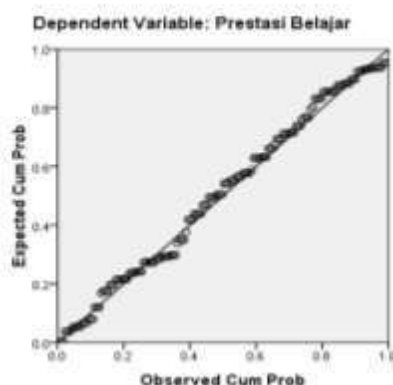
Gambar 2. Uji Normalitas
