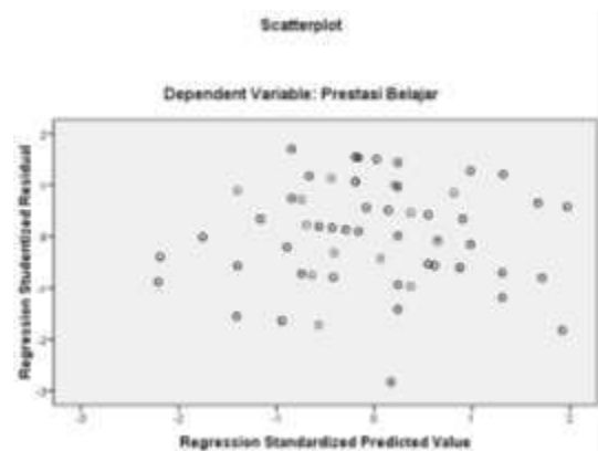
Gambar 3. Uji Heterokedastisitas
