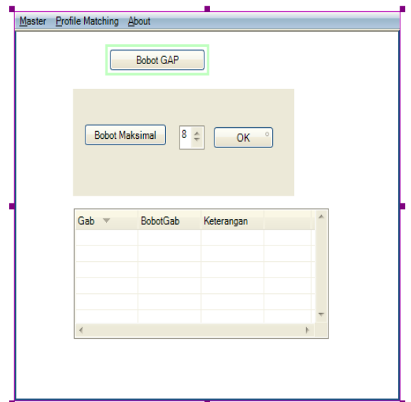
Gambar 3.19 Rancangan Tampilan Menu Tabel Daftar Gap
