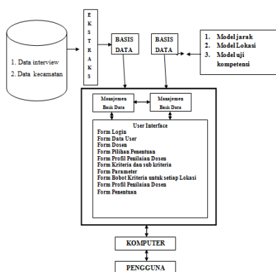
Gambar 3.1 Arsitektur SPK Penentuan Dosen pembimbing lapangan KKM
