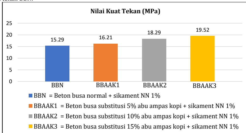
Gambar 5. Hubungan Kuat Tekan Beton Dengan Variasi Substitusi Abu Cangkang Kopi
