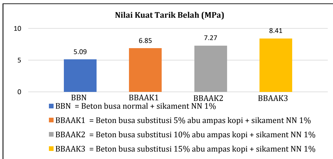
Gambar 6. Hubungan Kuat Tarik Belah Beton Dengan Variasi Substitusi Abu Cangkang Kopi Menggunakan Sikament NN
