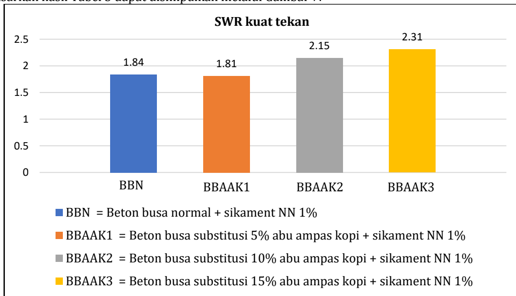
Gambar 7. SWR nilai kuat tekan
