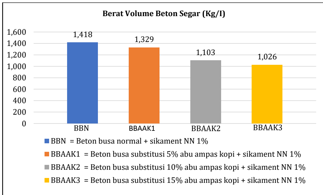
Gambar 4. Hubungan variasi substitusi abu cangkang kopi menggunakan sikament NN dengan berat volume beton segar.
