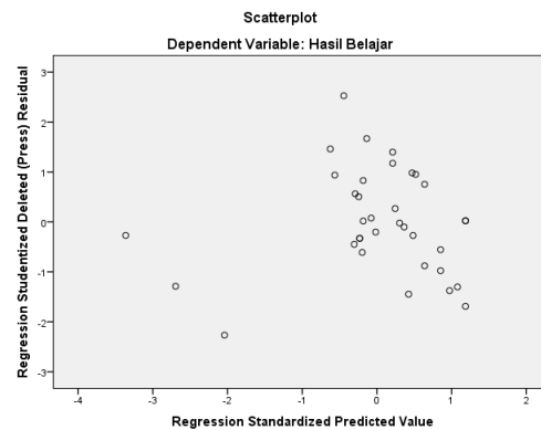
Gambar 3. Uji Heterokedastisitas
